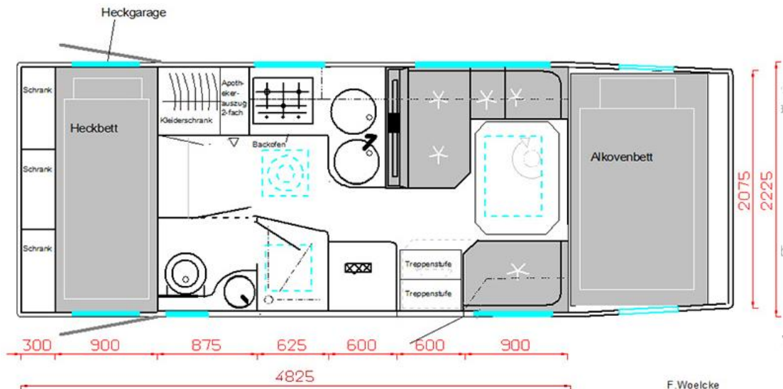
Grundriss
