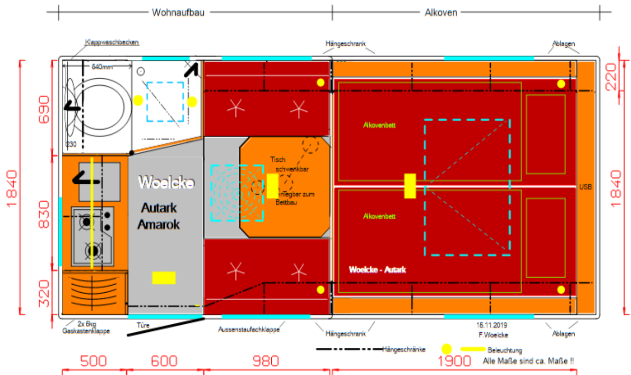
Der Grundriss
